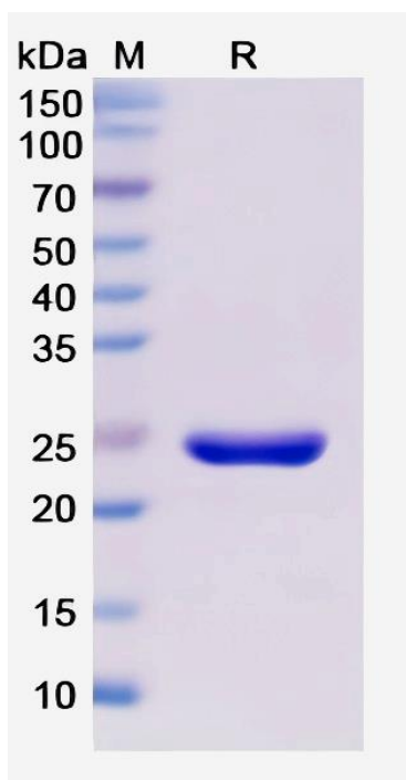
SDS-PAGE
