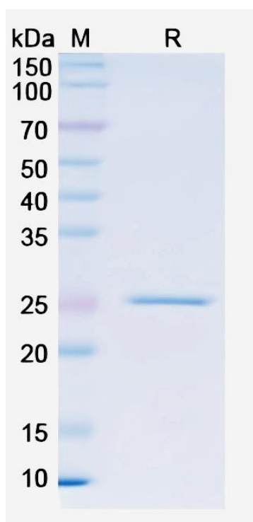
SDS-PAGE
