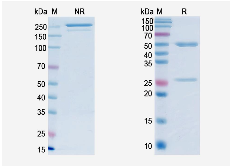
SDS-PAGE
