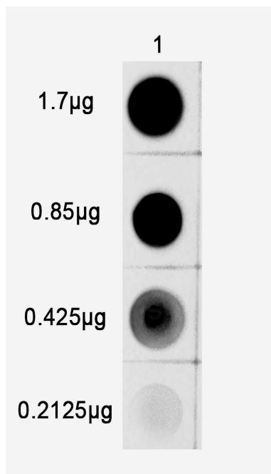
Dot Blot
